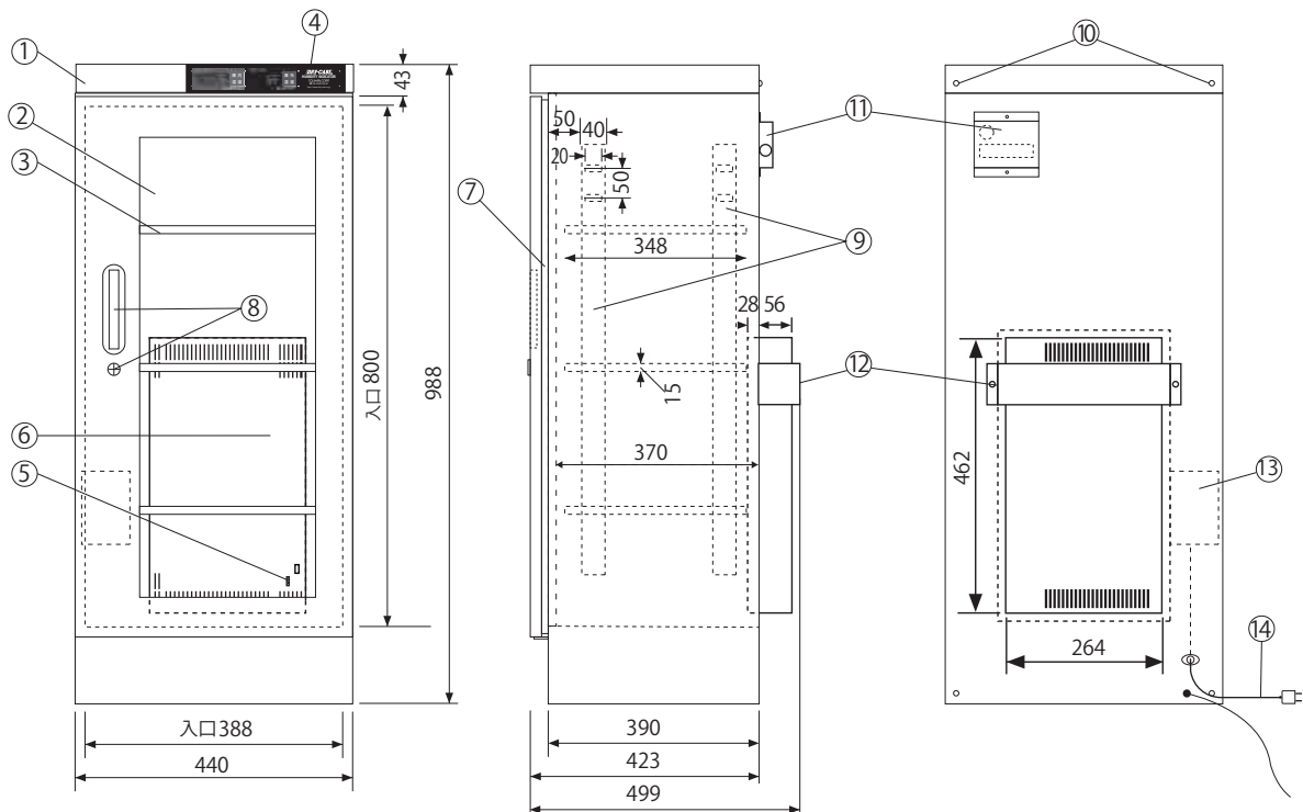
各部名称及び寸法 (mm)
