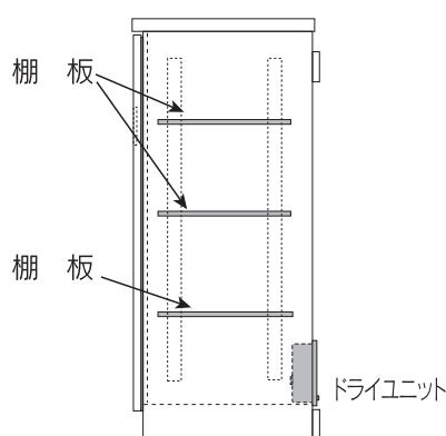
300 側面図
