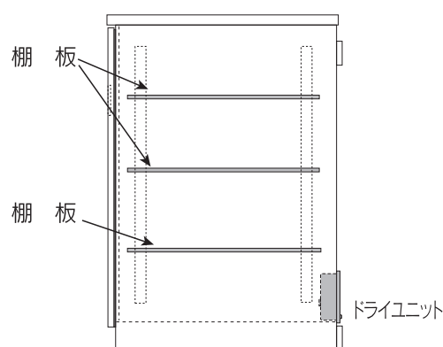
500 側面図
