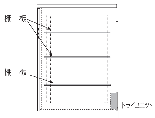
512 側面図
