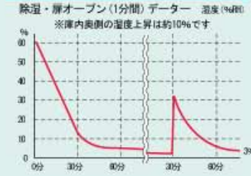
TDC-158-ADD 庫内湿度測定例
