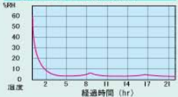
TDC-298-ADD 庫内湿度測定例
