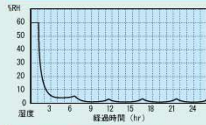
TDC-1419-SDD (%RH) 庫内湿度測定例
