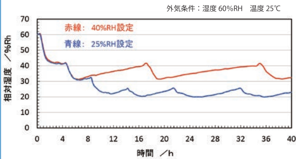
TDC-300-DX 庫内湿度測定例 湿度設定試験
