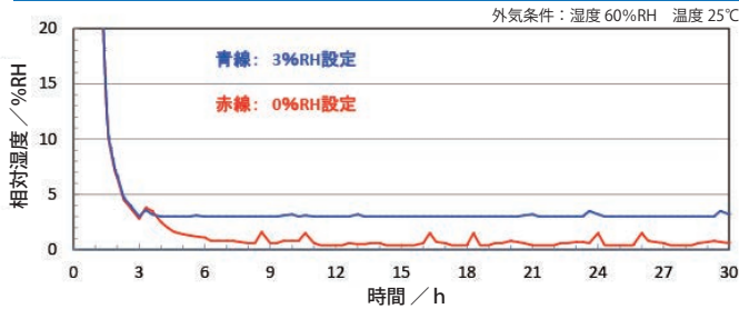
TDC-1300-HYP2 庫内湿度測定例 湿度設定試験
