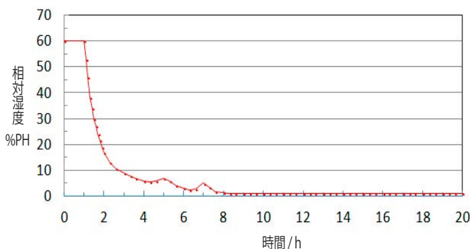
AC-250-LDX2 庫内湿度測定
