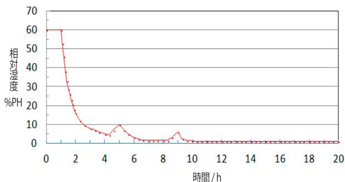
AC-110-LDX2 庫内湿度測定
