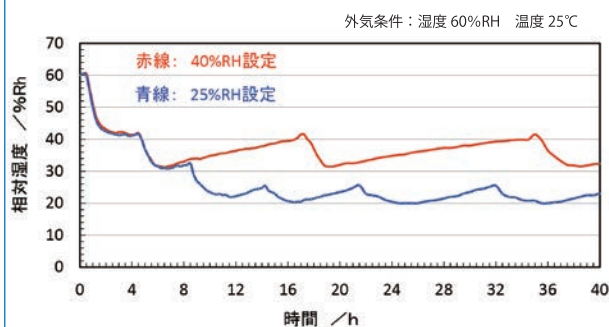
TDC-300-DX 庫内湿度測定例 湿度設定試験
