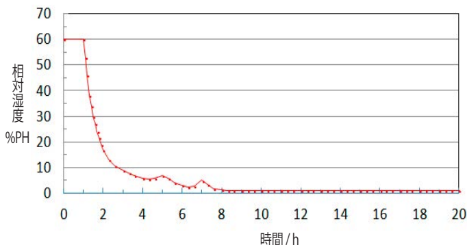
AC-252-LDX 庫内湿度測定
