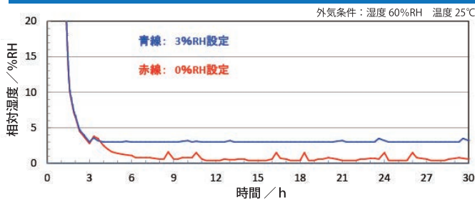
TDC-1332-HYP 庫内湿度測定例 湿度設定試験
