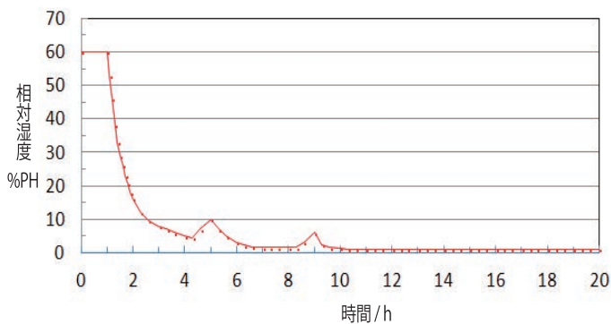
AC-110-LDX 庫内湿度測定
