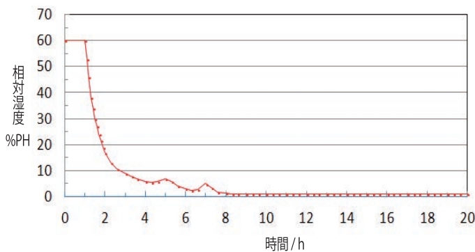
AC-250-LDX 庫内湿度測定
