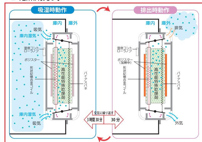
※2 乾燥剤方式
